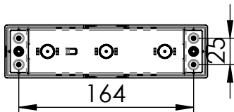
Bohrmaße
