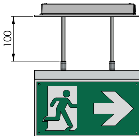
Deckenmontage mit 1x Zubehör (Art. Nr.: 660010970) "Verlängerung Deckenabstand 10 cm"
