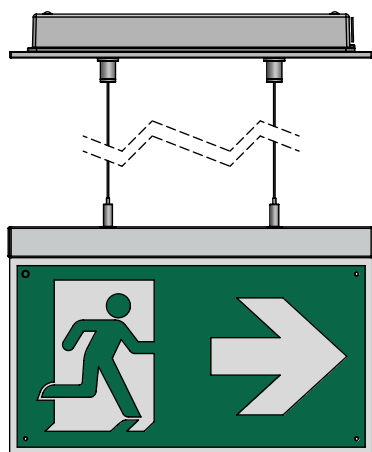
Deckenmontage mit 1x Zubehör (Art. Nr.: 660010910)) "Seilmontage 1500mm"
