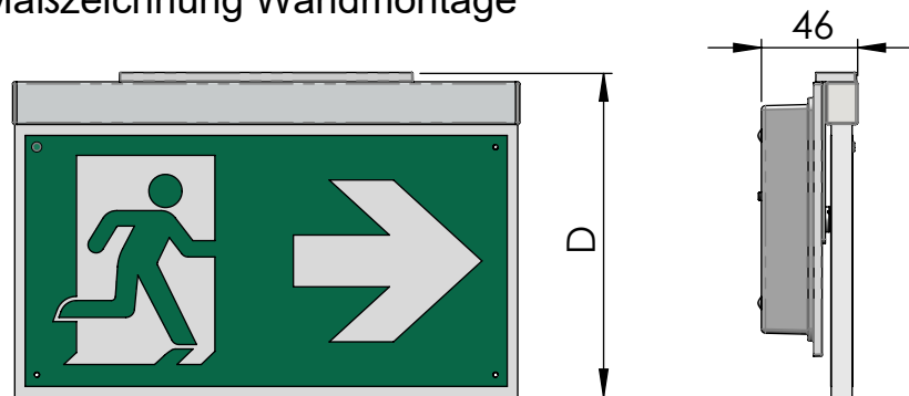
Maßzeichnung Wandmontage
