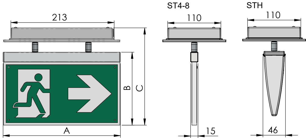
Maßzeichnung Deckenmontage
