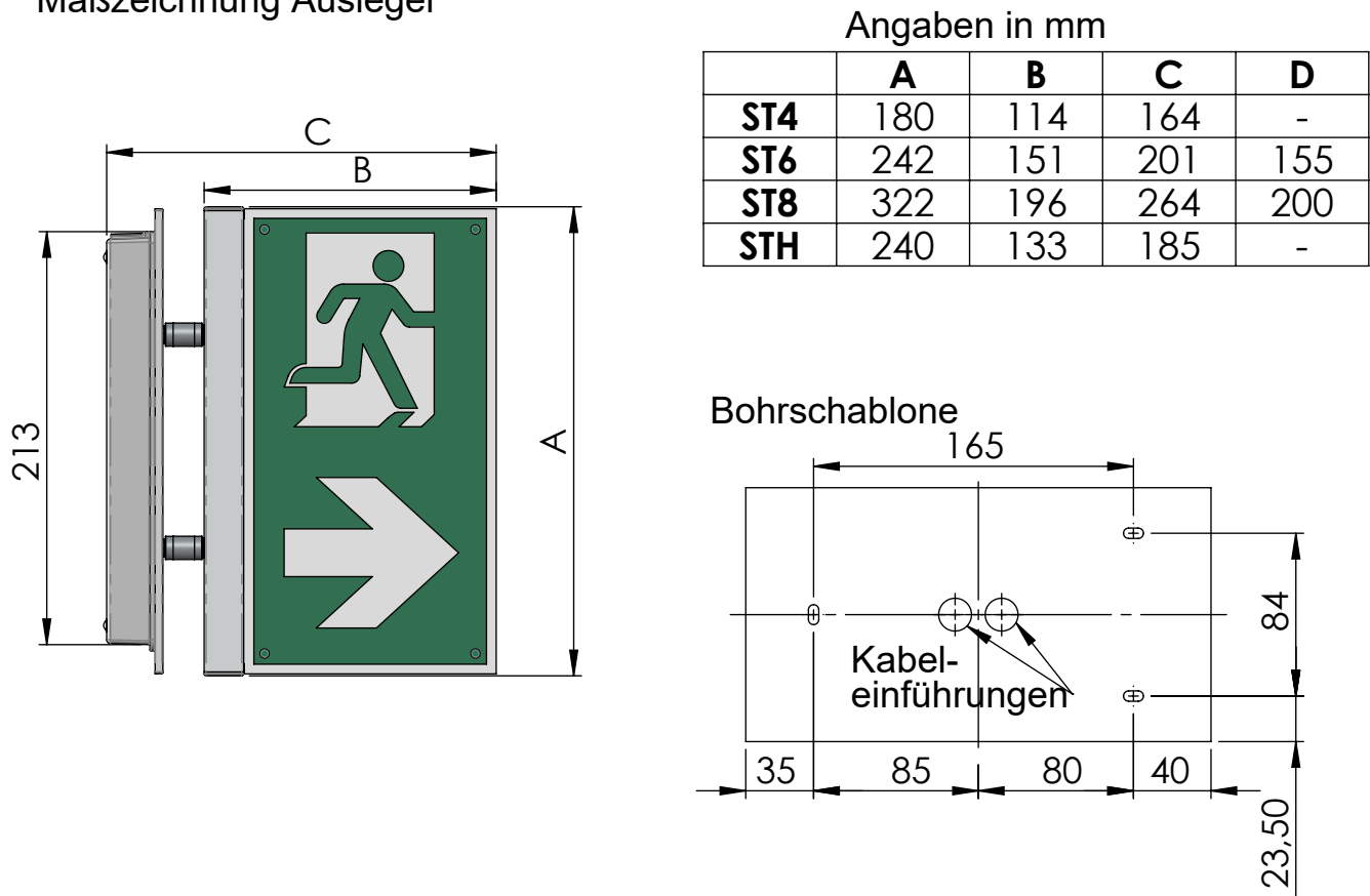
Maßzeichnung Ausleger
