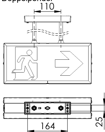
Doppelpendel
