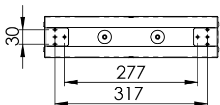
Deckenmontage Abstand
