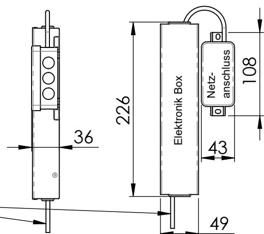
Zentralbatterie mit Überwachungsbaustein
