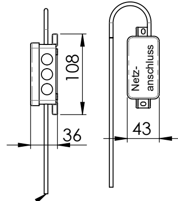
Zentralbatterie E-220
