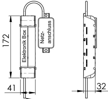
Einzelbatterie AX-Version
