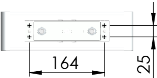
Bohrmaße
