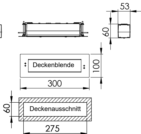
Deckeneinbau
