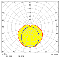
UL3-D = Deckenmontage (hohe Haube D) ohne Pikto
