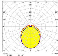
UL3-WD = Deckenmontage (flache Haube WD) ohne Pikto
