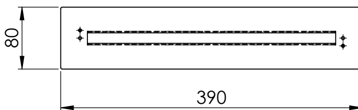
Deckeneinbaublende
